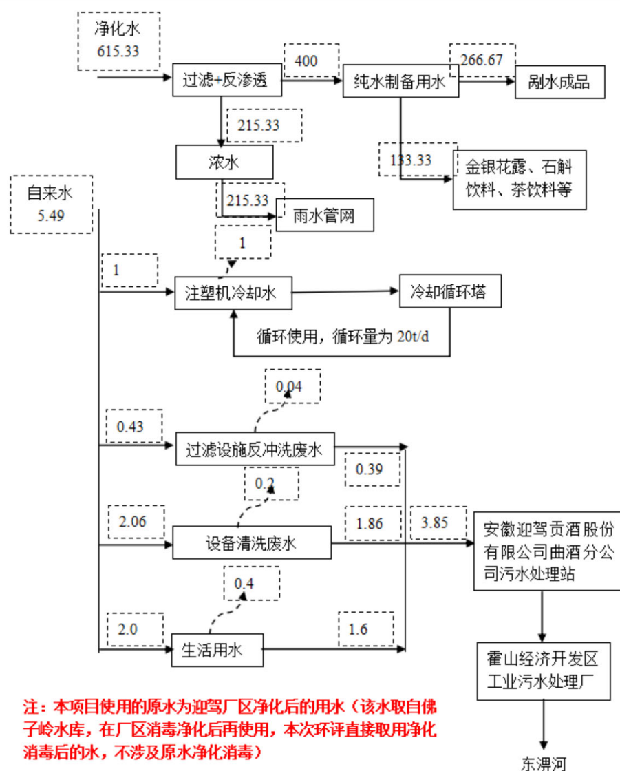
图 用水平衡图（t/d）
