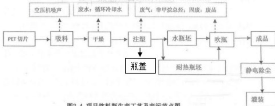
图2.4 项目饮料瓶生产工艺及产污节点图
